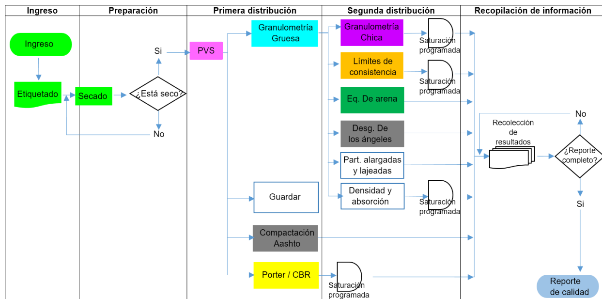
Figura 3. Diagrama de flujo de la línea de trabajo de terracerías y materiales pétreo
